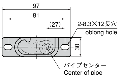
(キーパーL) Keeper
