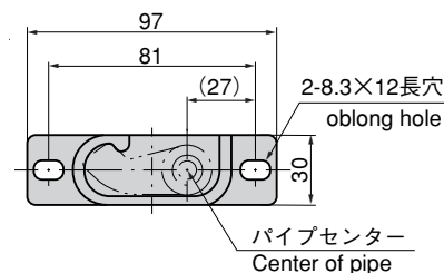
(キーパーL) Keeper
