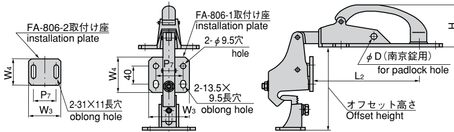
〔ハンドル本体〕 Handle main body
