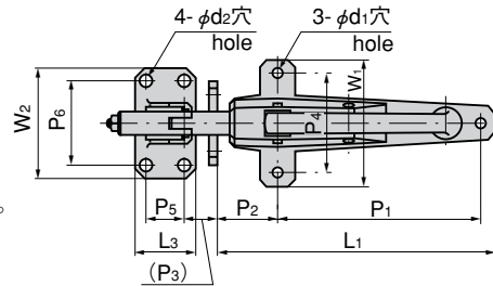
カギピン Key pin
