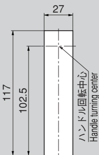
パネル穴明け寸法 Panel drilling dimensions
