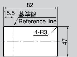
パネル穴明け寸法 (A-542-4-R) Panel drilling dimensions
