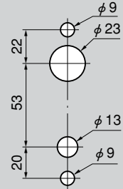
パネル穴明け寸法 Panel drilling dimensions
