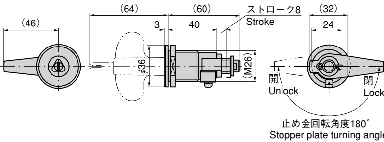
[A-169-1 本体] Main body
