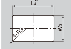
パネル穴明け寸法 Panel drilling dimensions
