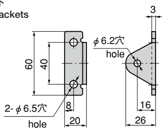
B-461-2~4用 標準ブラケット [B-461-A-2] Standard brackets
