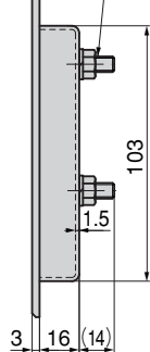
2-M6×20 六角ボルト hexagon head bolt
