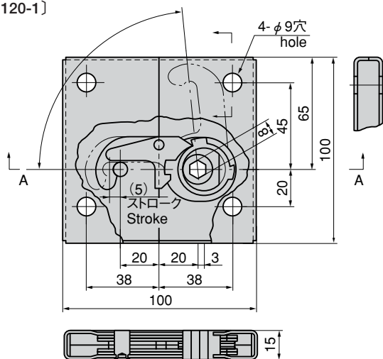
A-A 断面 Cross section
