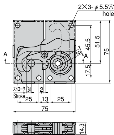
A-A 断面 Cross section
