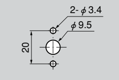
パネル穴明け寸法 Panel drilling dimensions
