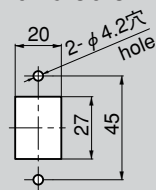
本体パネル穴明け寸法 Main panel drilling dimensions
