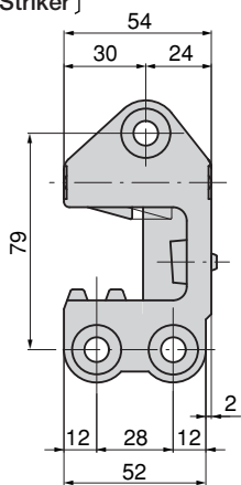
〔受金具 Striker〕
