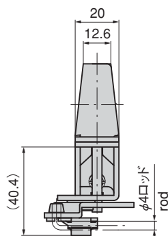
使用ロッド接続部加工図 Figure of machining rod for connection
